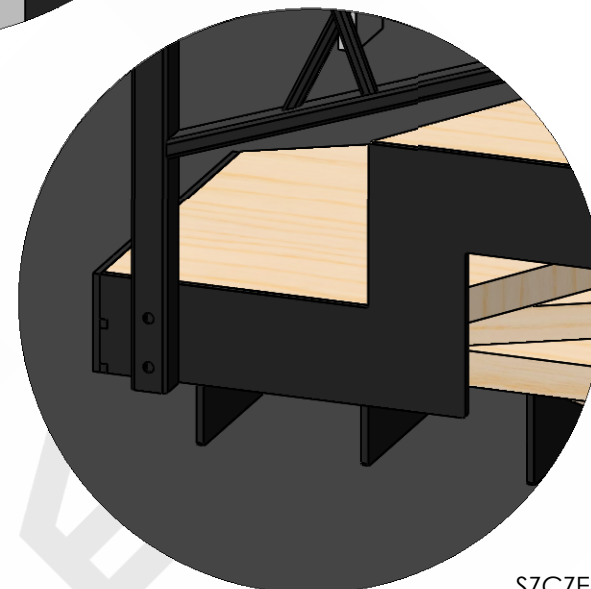
SZCZEGÓŁ B SKALA 1 : 8
