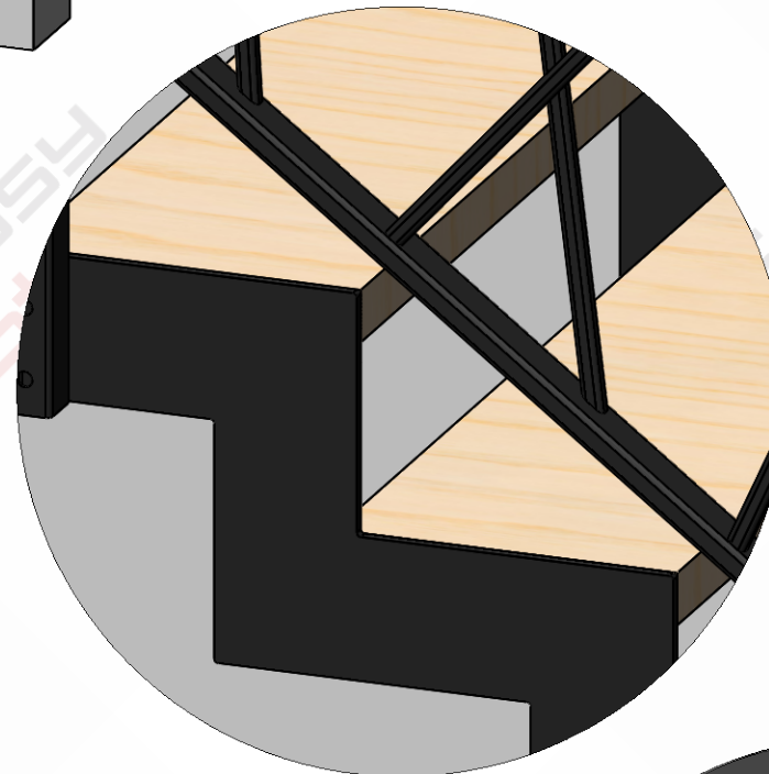
SZCZEGÓŁ C SKALA 1 : 6
